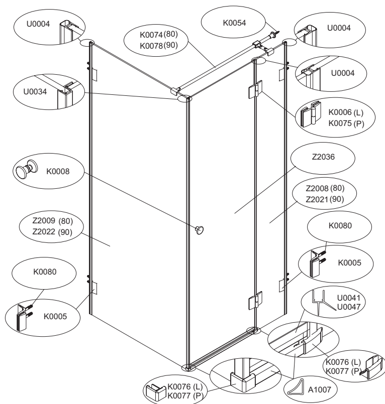
Na rysunku przedstawiono kabinę w wersji prawej
